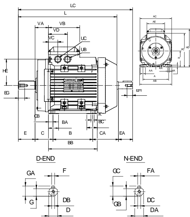
Motor con patas; IM B3 (IM 1001), IM 1002
