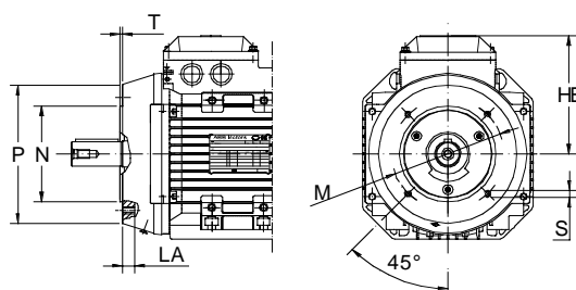
Motor con brida pequeña; IM B14 (IM 3601)
