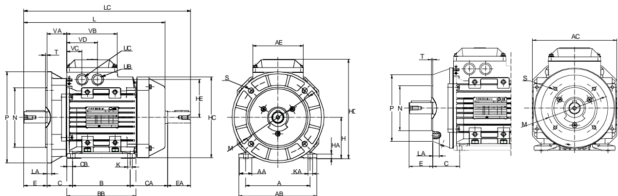
Motor con patas y brida; IM B35 (IM 2001), IM 2002, brida grande
