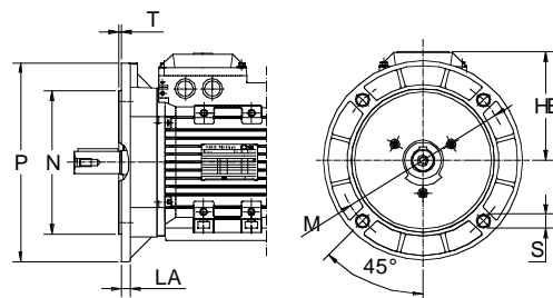
Motor con brida pequeña; IM B14 (IM 3601)
